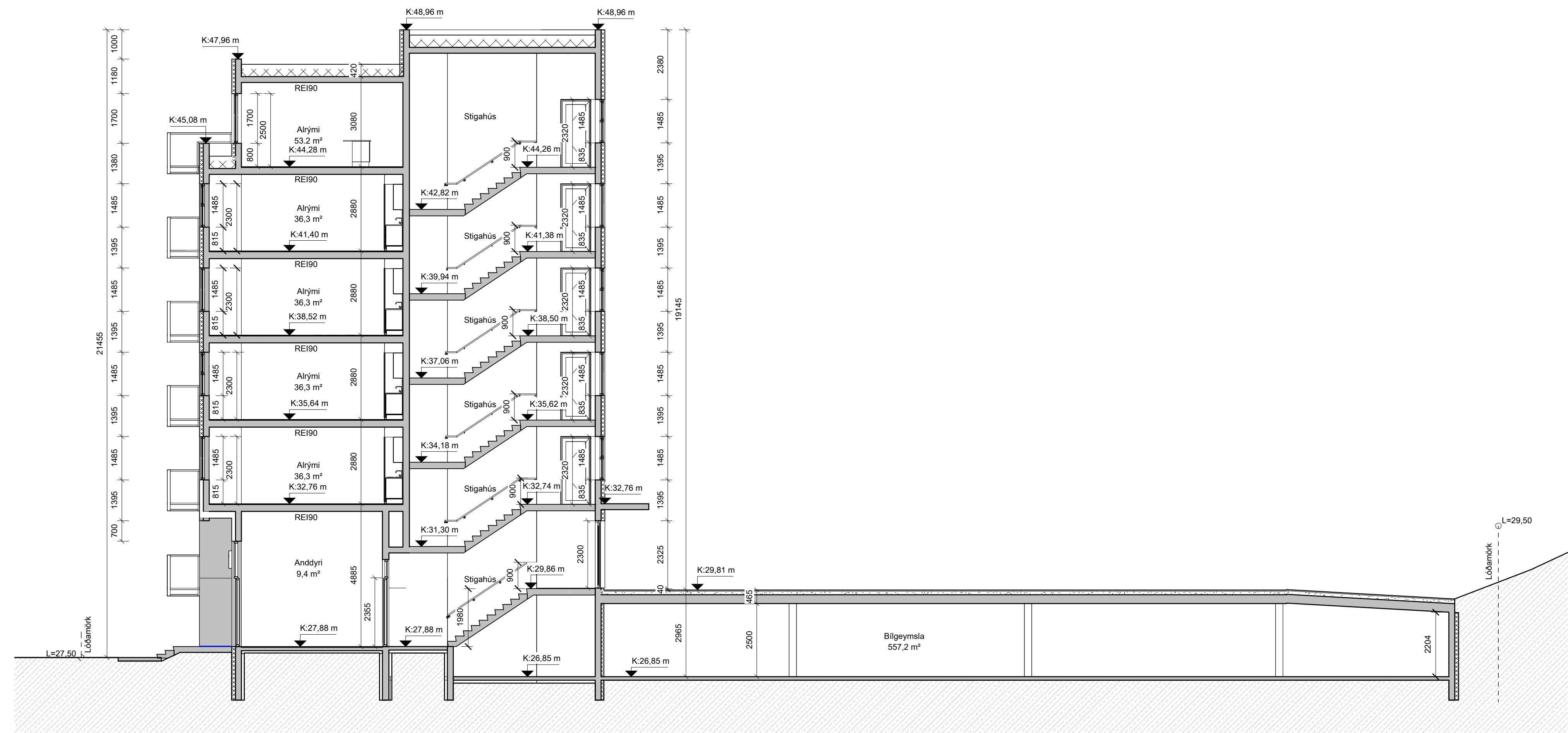
Snið C-C mkv: 1 : 100
