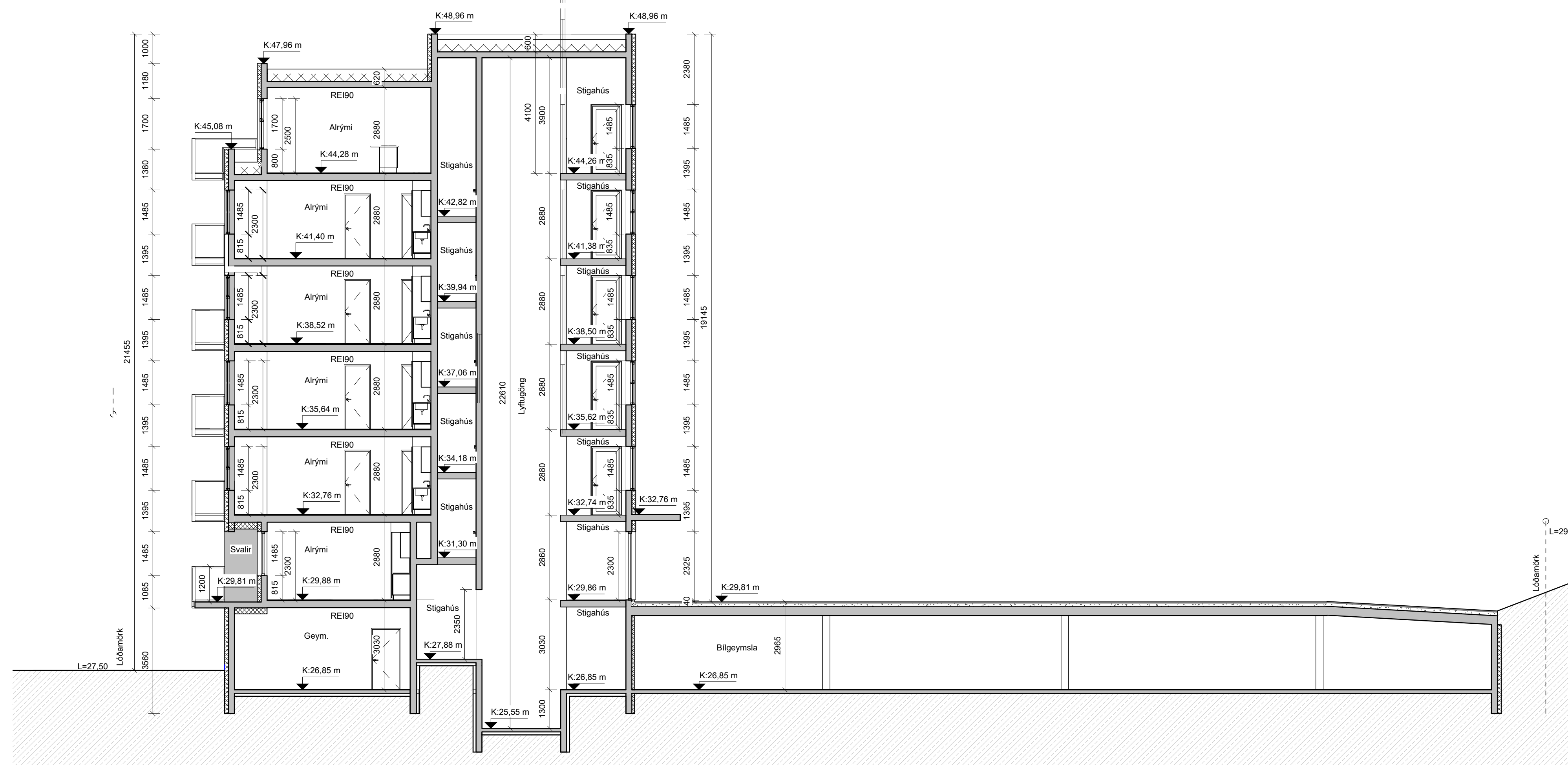
Snið B-B mkv: 1 : 100
