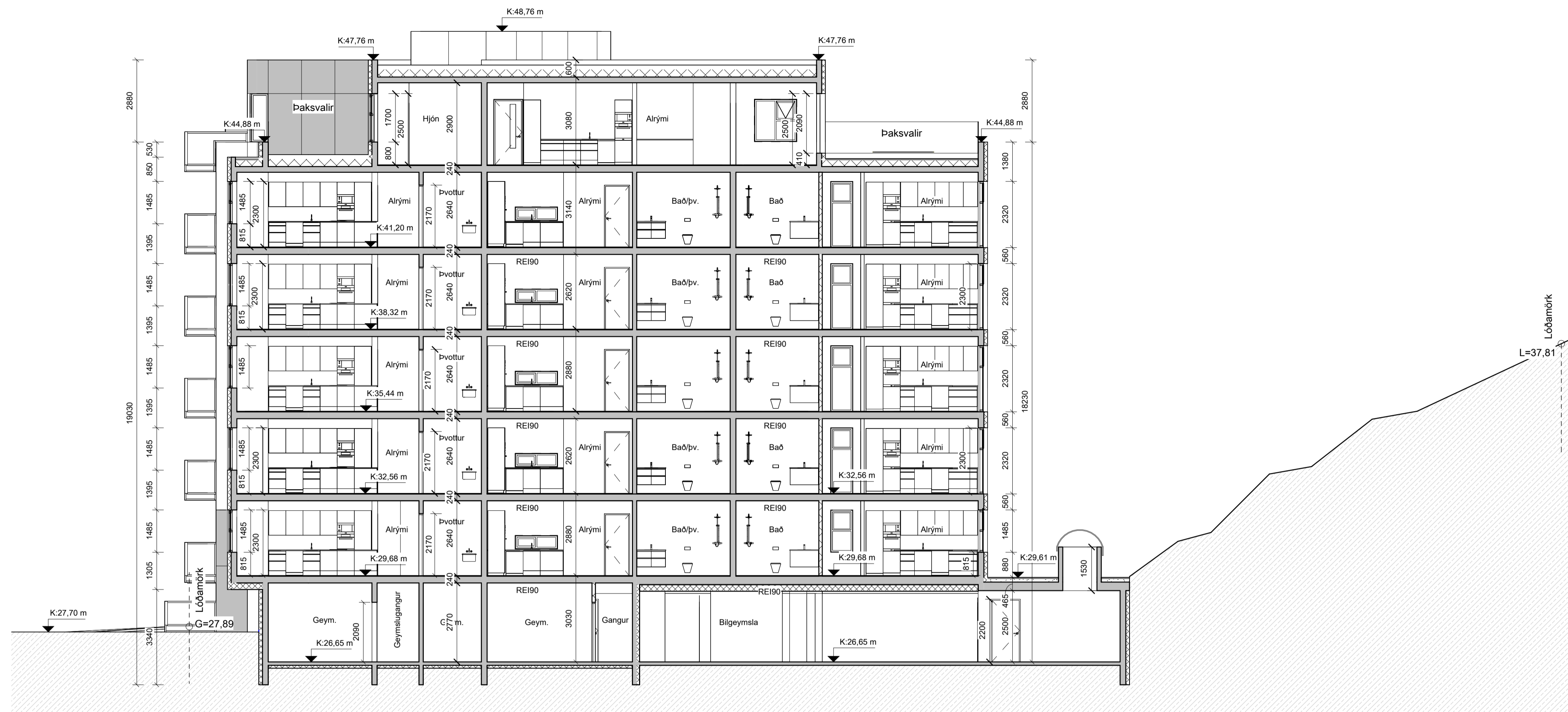
Snið C-C mkv: 1 : 100
